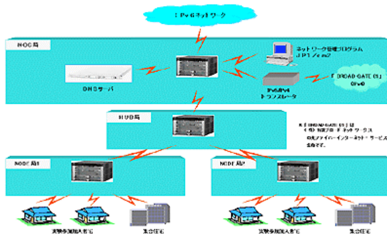
usen の IPv6 実験ネットワーク構成図
